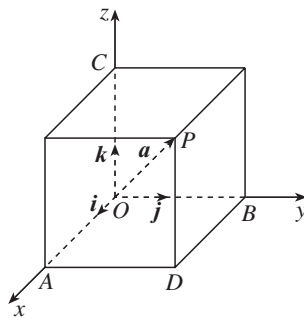
图 10 向量标准正交分解
