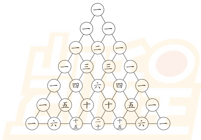
图 12 杨辉三角
